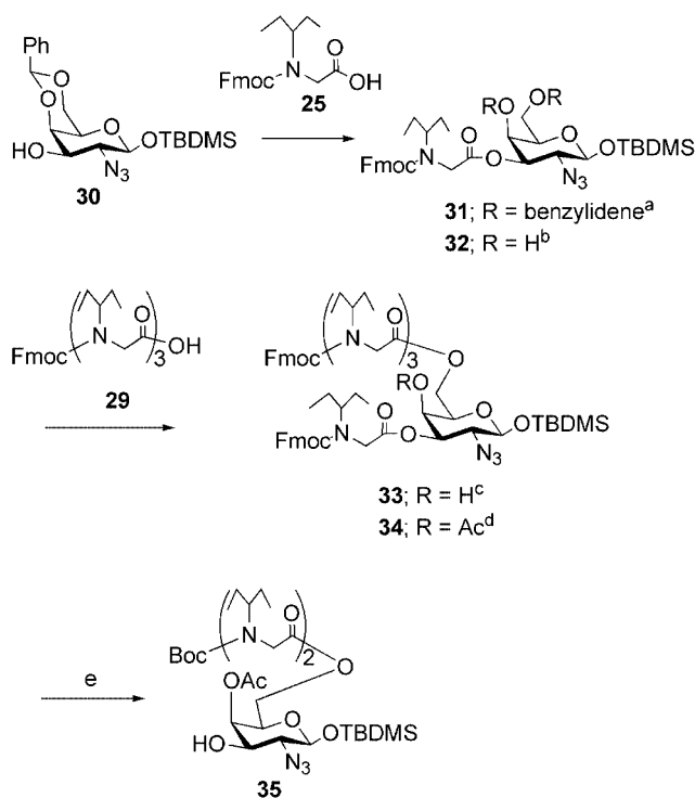
Scheme 4. Reagents and conditions. a 25 , cyanuric chloride, pyr., 40 °C, 2 h, 90%; b 80% aq. AcOH, 60 °C, 2 h, 79%; c 29 , cyanuric chloride, pyr., 40 °C, 2 h, 65%; d Ac 2 O, pyr., 40 °C, 2 h, 91%; e i), 20% piperidine in DMF, room temp., 20 min. ii), PTC, NMM, room temp., 30 min. iii), TFA, CH 2 Cl 2 , room temp., 30 min. iv), Boc 2 O, satd. aq. NaHCO 3 , DMF, room temp., 30 min, 69% (4 steps).
